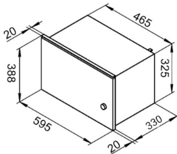
Размеры прибора
