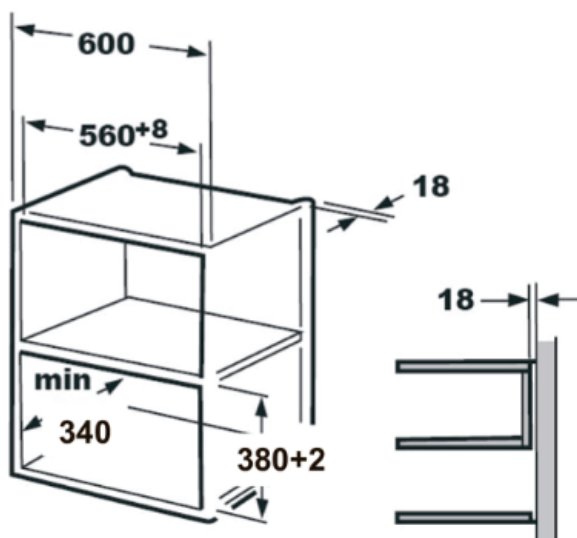
Установка СВЧ в нишу
