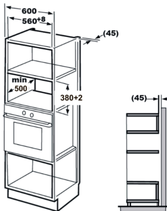
Установка СВЧ в нишу над духовым шкафом
